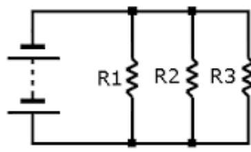
CIRCUITO PARALELO
